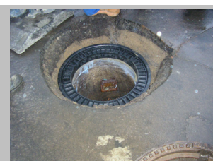
3. Auflegen des ersten Ringes auf das Mörtelbett
