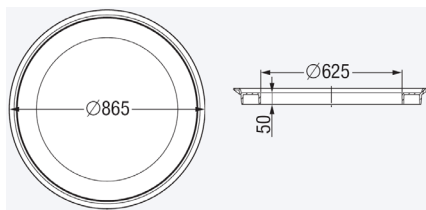
KESSEL-Ausgleichsring 860147
