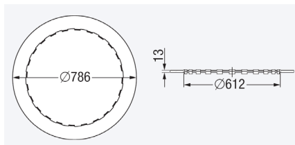
KESSEL-Ausgleichsring 860147
