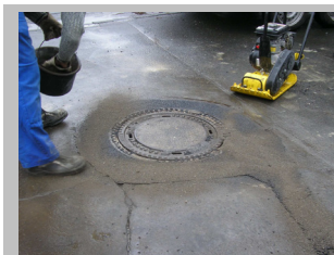
13. Abstreuen mit Bruchsand oder Schamott
