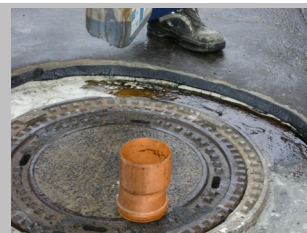
10. Aufbringen eines Haftklebers oder einer polymermodifizierten Bitumenemulsion
