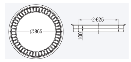
KESSEL-Ausgleichsring 860149
