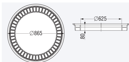
KESSEL-Ausgleichsring 860148
