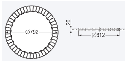
KESSEL-Ausgleichsring 860148
