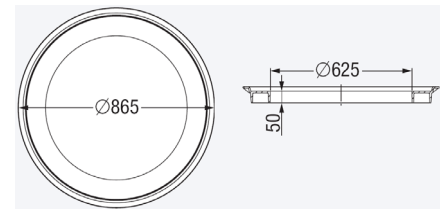
KESSEL-Ausgleichsring 860149
