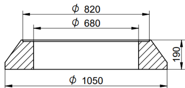
Schnitt A-A
