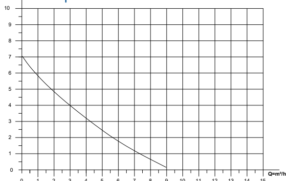
H=m Pumpenkennlinie
