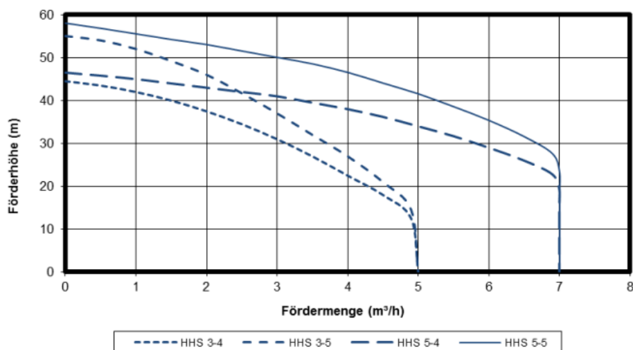
Pumpenkennlinie
