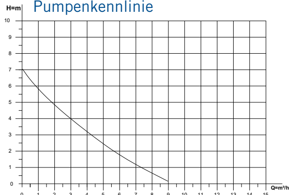
Pumpenkennlinie
